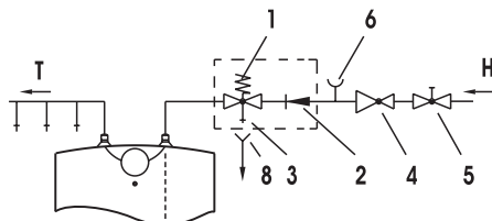
Montage under tvättstället
