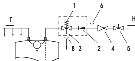
Alsó elhelyezésű kivitel
