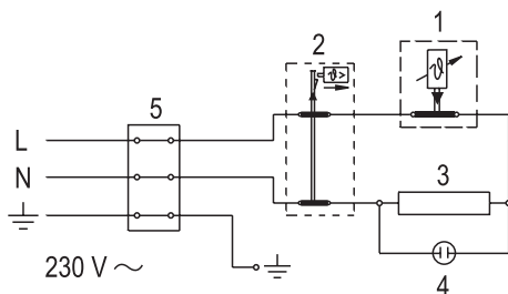
Шема електричног вязала
