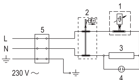
Az elektromos kapcsolás vázlata
