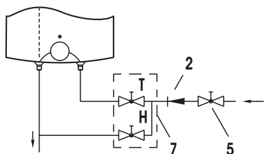
Montage ovanför tvättstället
