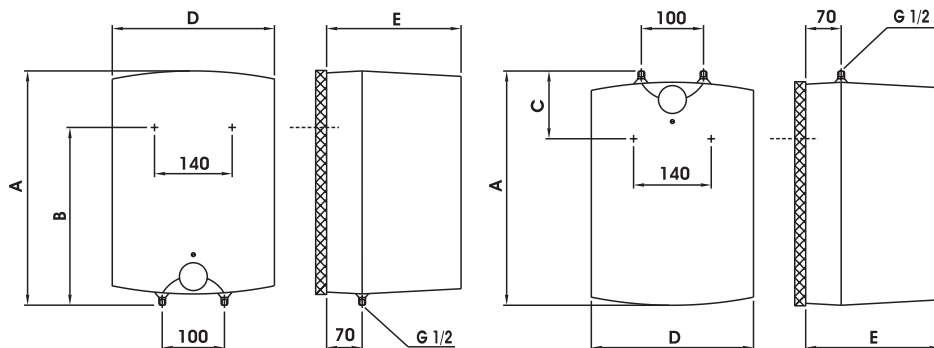
Uitvoering voor montage boven de wastafel Uitvoering voor montage onder de wastafel
